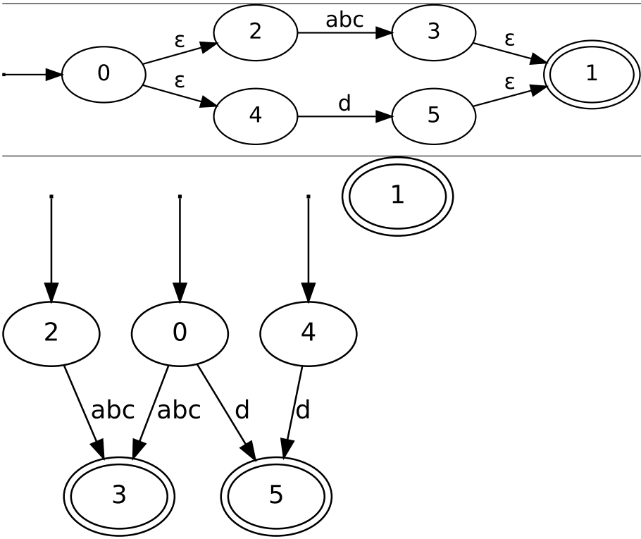
Рис. 2.3: «NFAs for «abc|d»)
