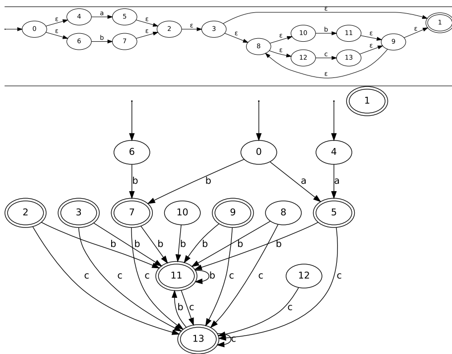
Рис. 2.4: «NFAs for «(a|b)(b|c)*»)
